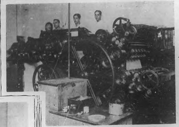
La rotative donde se imprimen los billetes. Mr. Gustavo Eriksson, (que no aparece en la foto), es el Jefe del Departamento de Máquinas.
